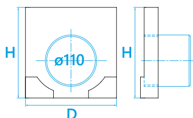
Ścianka czołowa z króćcem
